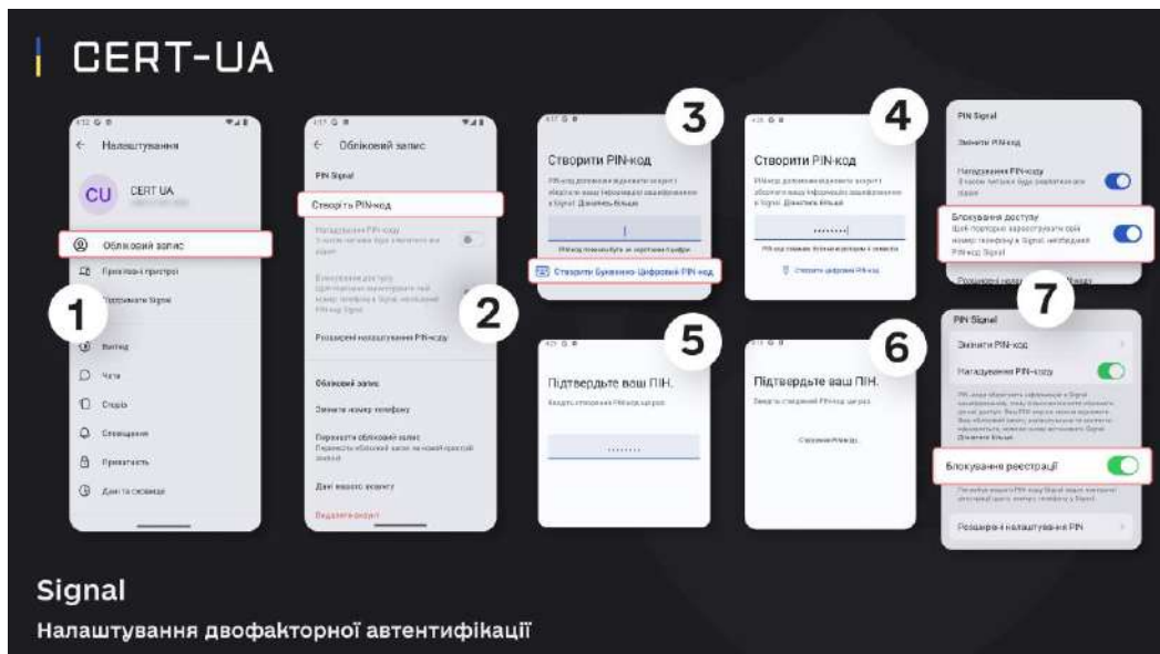
Рис.4 Налаштування 2FA в Signal
